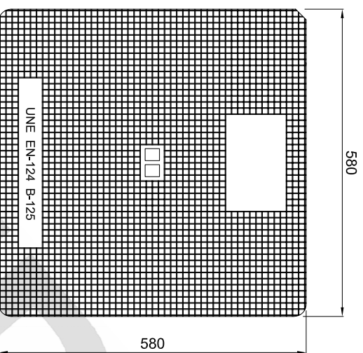
TAPA. VISTA SUPERIOR.
