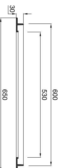
MARCO. SECCIÓN.
